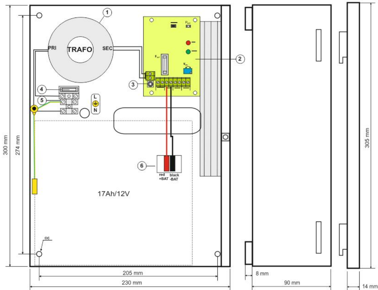
Fig. 3. Vedere interior sursă de alimentare.
