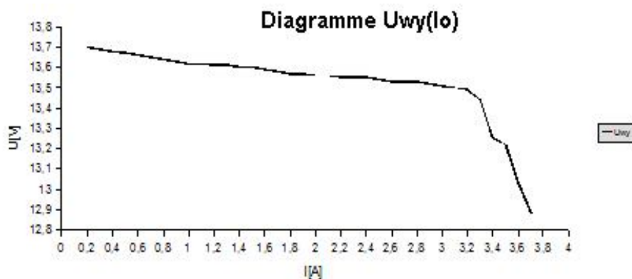
Fig. 4. Caracteristica curent-tensiune a sursei de alimentare.
