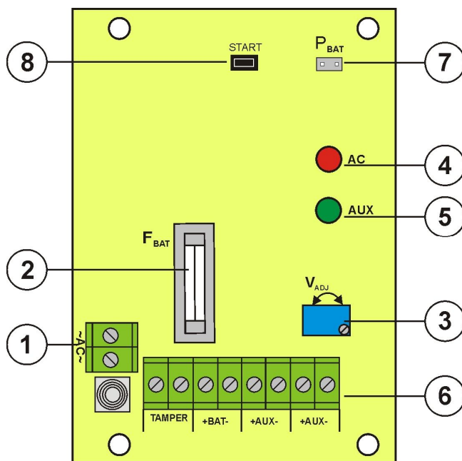
Fig. 2. Vedere placă de bază.
