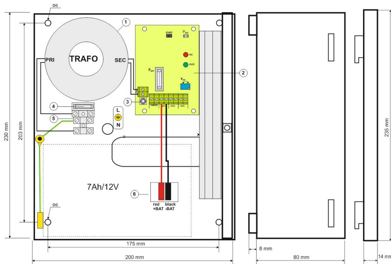
Fig. 3. Vedere interior sursă de alimentare.
