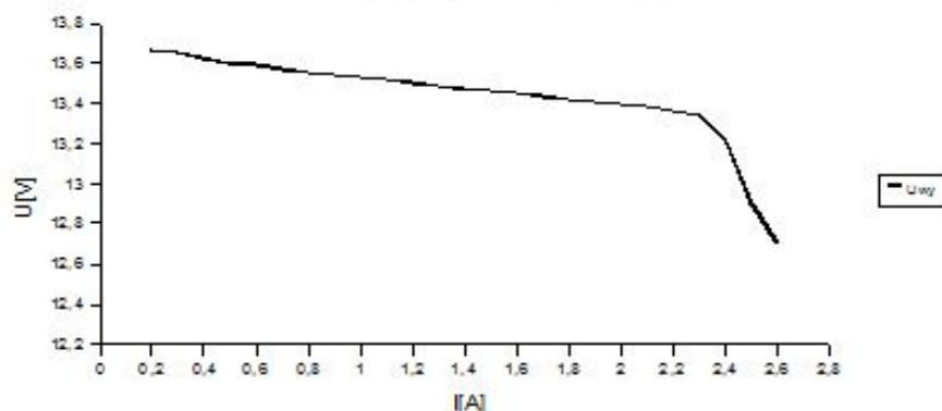
Fig. 4. Caracteristica curent-tensiune a sursei de alimentare.
