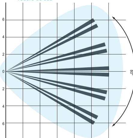
XDTP200H, XDTP200HM, - vedere de sus
